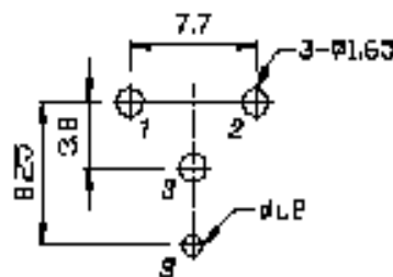
P.C.B LAYOUT(±0.1) (BOTTOM VIEW)
