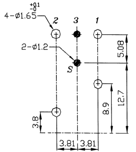
P.C.B LAYOUT(±0.1) (BOTTOM VIEW)
