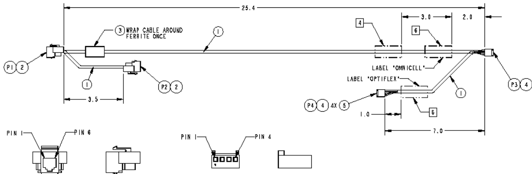
ITEM 2 SCALE 1:1
